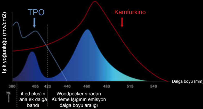
iLed plus Spektral Eğrisi ve Reçine Spektral Soğurma
